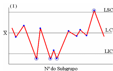
FIGURA 01 - Gráfico de controle \bar{X} fora de controle
