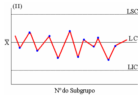
FIGURA 02 - Gráfico de controle \bar{X} sob controle
