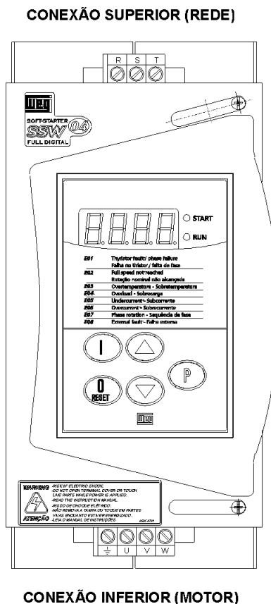
FIG. 3.5 - Localização das conexões de potência/aterramento
