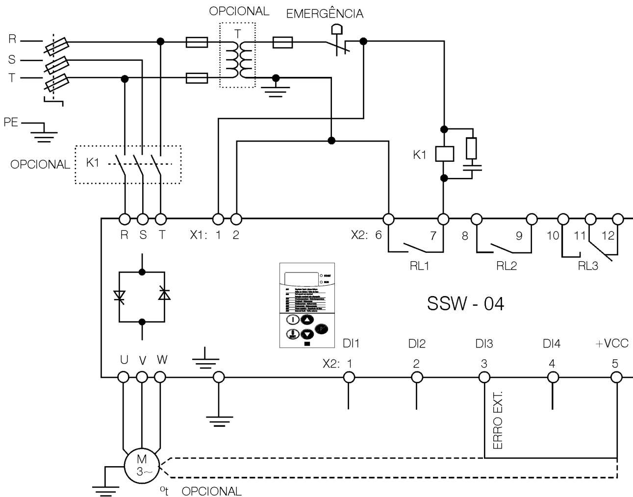
Figura 3.7 - Conexões mínimas para operações pela IHM.
